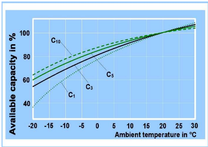
Доступная емкость в зависимости от температуры.
