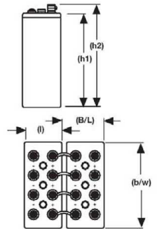
20 OPzV 2500 – 24 OPzV 3000
