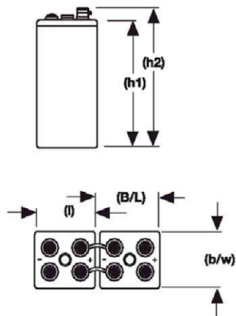
8 OPzV 800 – 12 OPzV 1500
