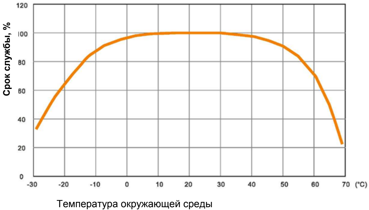
Зависимость срока службы от температуры окружающей среды
