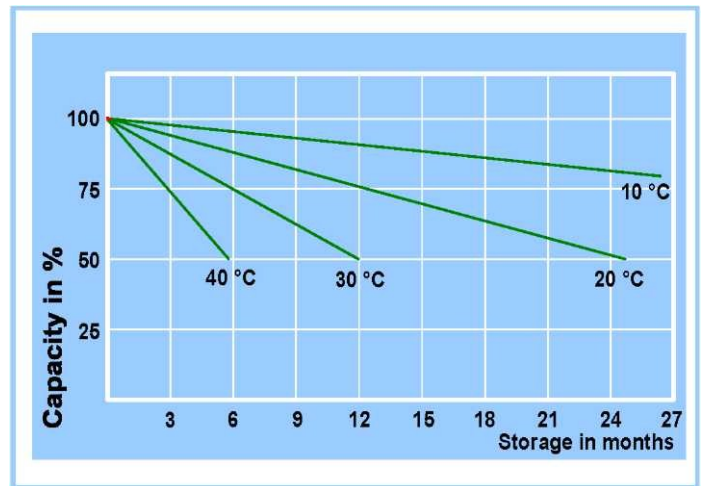
Саморазряд и остаточная емкость
