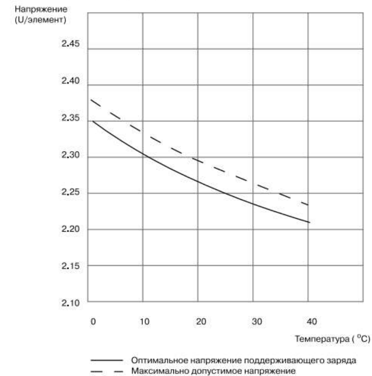
Напряжение поддерживающего заряда в зависимости от температуры
